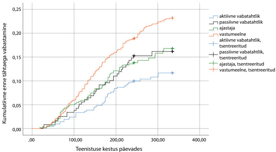
Joonis 3. Ajateenistusest enne tähtaega reservi arvamise kumulatiivne risk ajateenistusse astumise ja meelestatuse tüübi alusel 34
