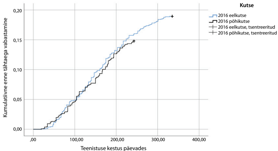
Joonis 2. Ajateenistusest enne tähtaega reservi arvamise kumulatiivne risk 33
